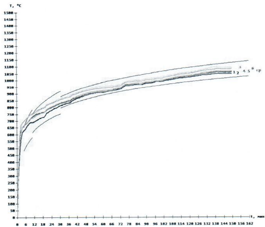
График изменения температуры в объеме испытательной печи при испытании образца № 2
